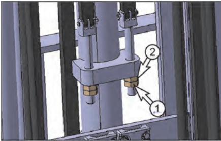
FFT 마스트 캐리지 체인의 보기
